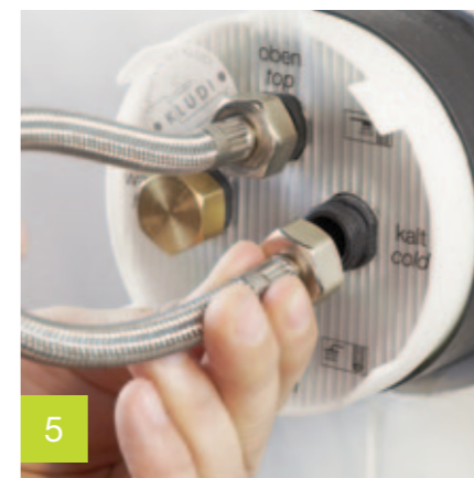
5 Propláchnutí podle DIN 1988 zabudovanou proplachovací sadou – bez otevření boxu
