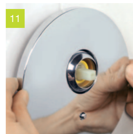
11 Nasadit bezzávitovou rozetu
