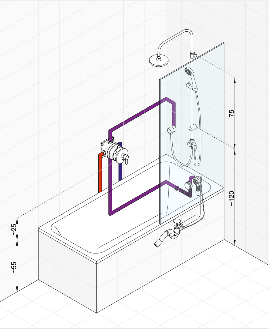
Napouštění vany přepadem. Vanová a sprchová baterie umožňuje přepínat vodu mezi napouštěním vany přepadem a KLUDI DUAL SHOWER SYSTÉMEM, který umí přepínat vodu mezi hlavovou a ruční sprchou.
