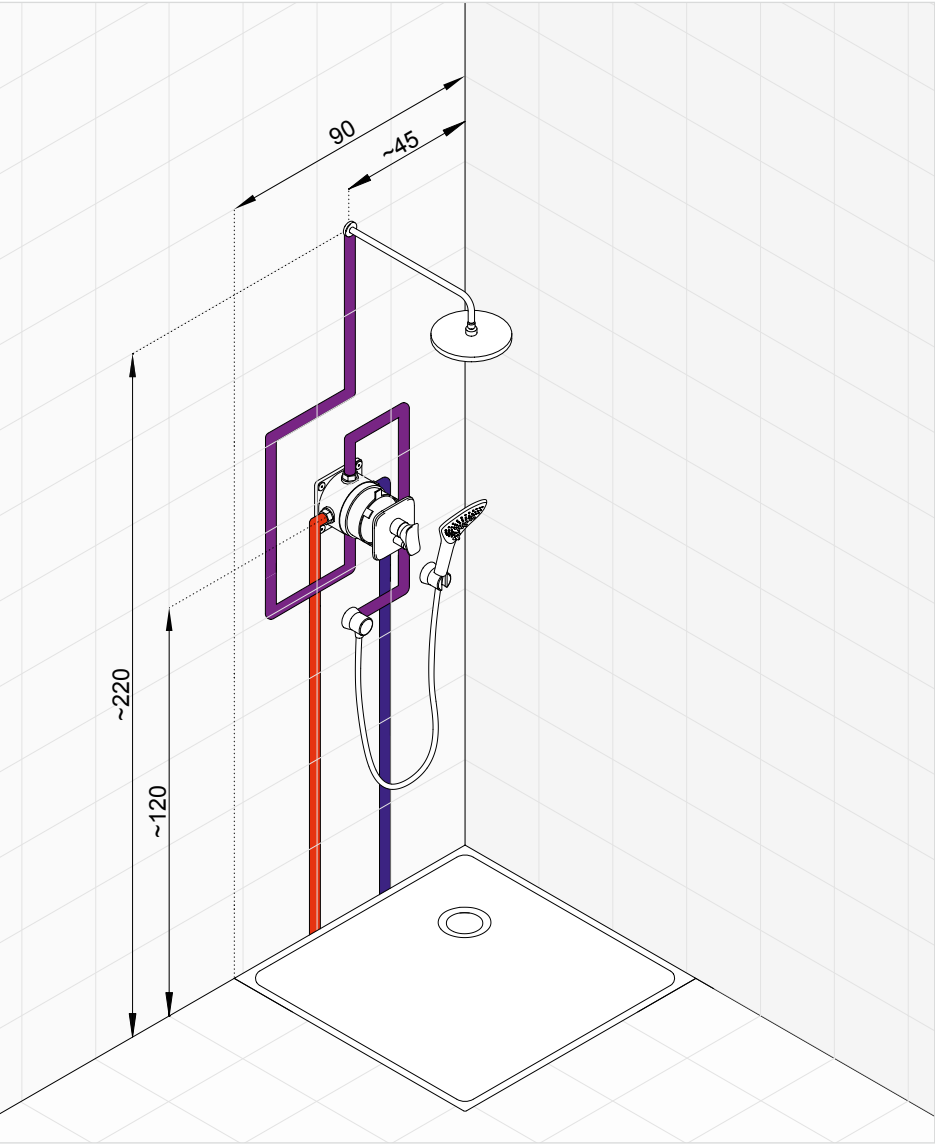
Klasická sestava podomítkové baterie pro hlavovou a ruční sprchu. Získáme dva sprchové vývody vody a všechno je ovládané jednou podomítkovou baterií s přepínačem.
