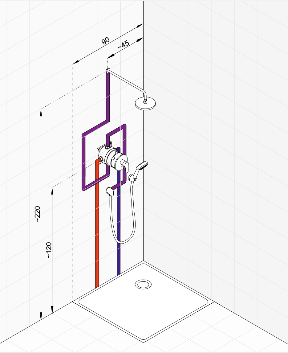
Klasický rozvod podomítkové baterie pro hlavovou a ruční sprchu. Získáme dva zdroje vody, vše je ovládáno podomítkovou baterií s přepínačem.
