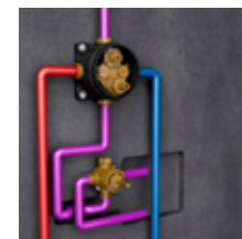
KLUDI - Instalace podomítkového rozvodu - sprcha Podomítková termostatická vanová a sprchová baterie, hlavová sprcha, boční trysky a ruční sprcha
