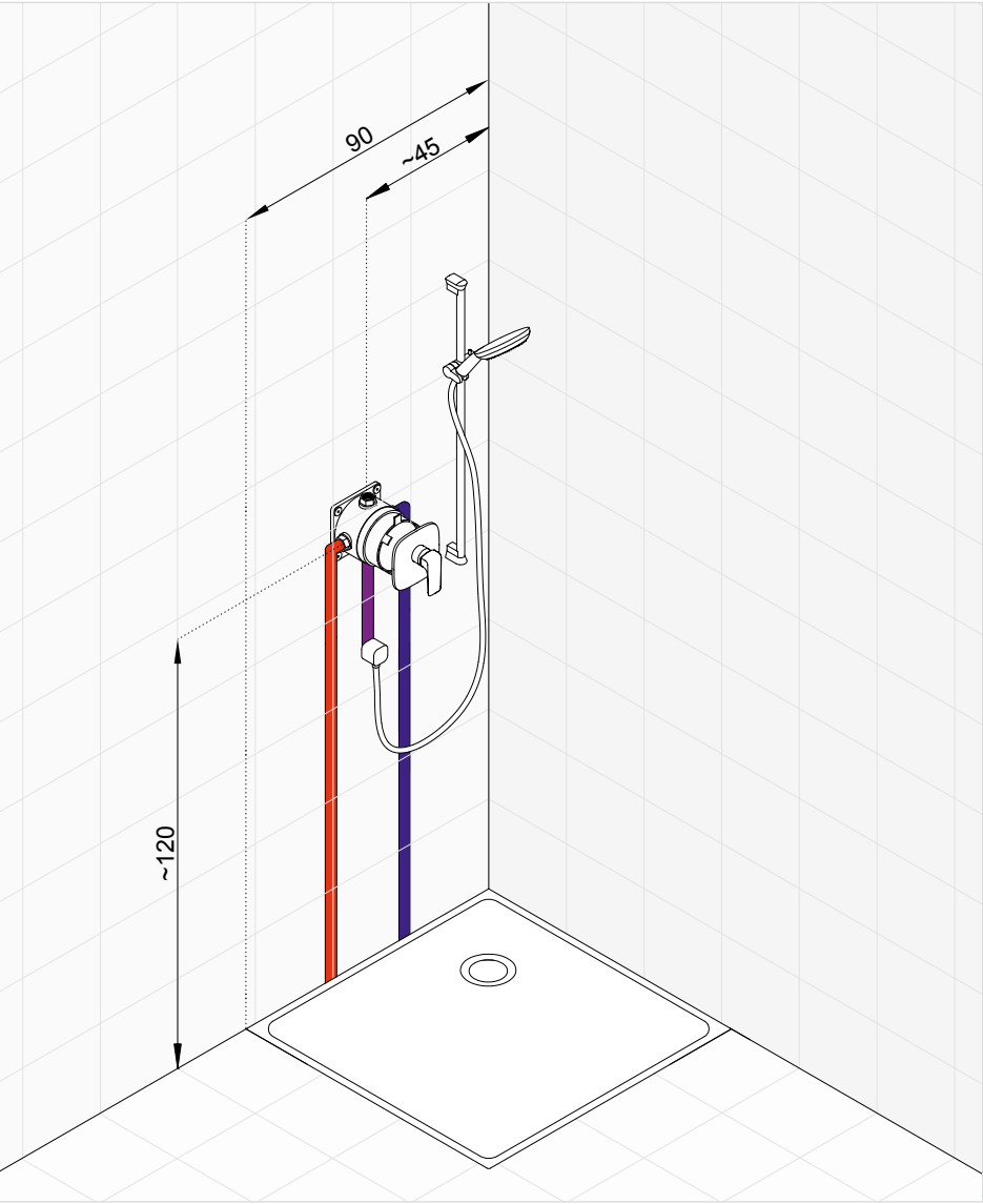
Klasický podomítkový rozvod ke sprchové soupravě.
