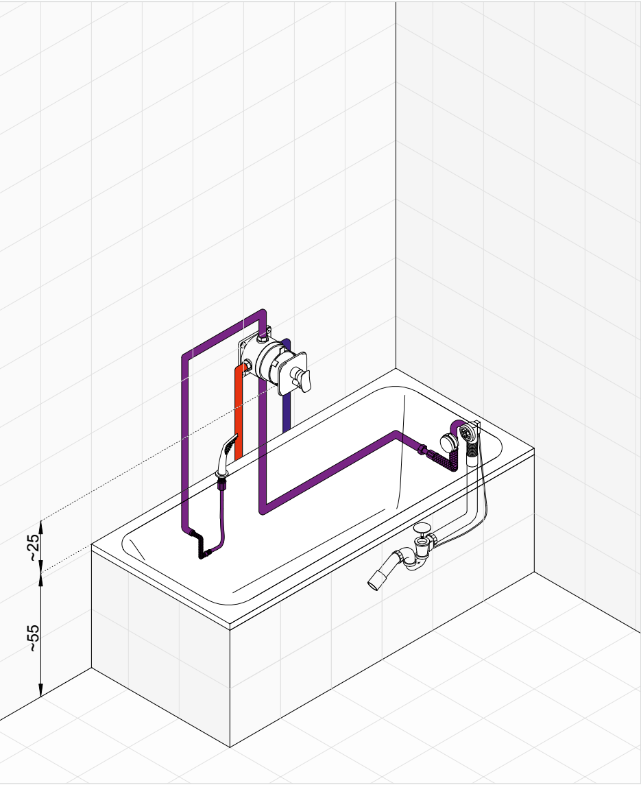
Napouštění vany přepadem. Vanová a sprchová baterie umožňuje přepínání vody do sprchové soupravy namontované na okraji vany.
