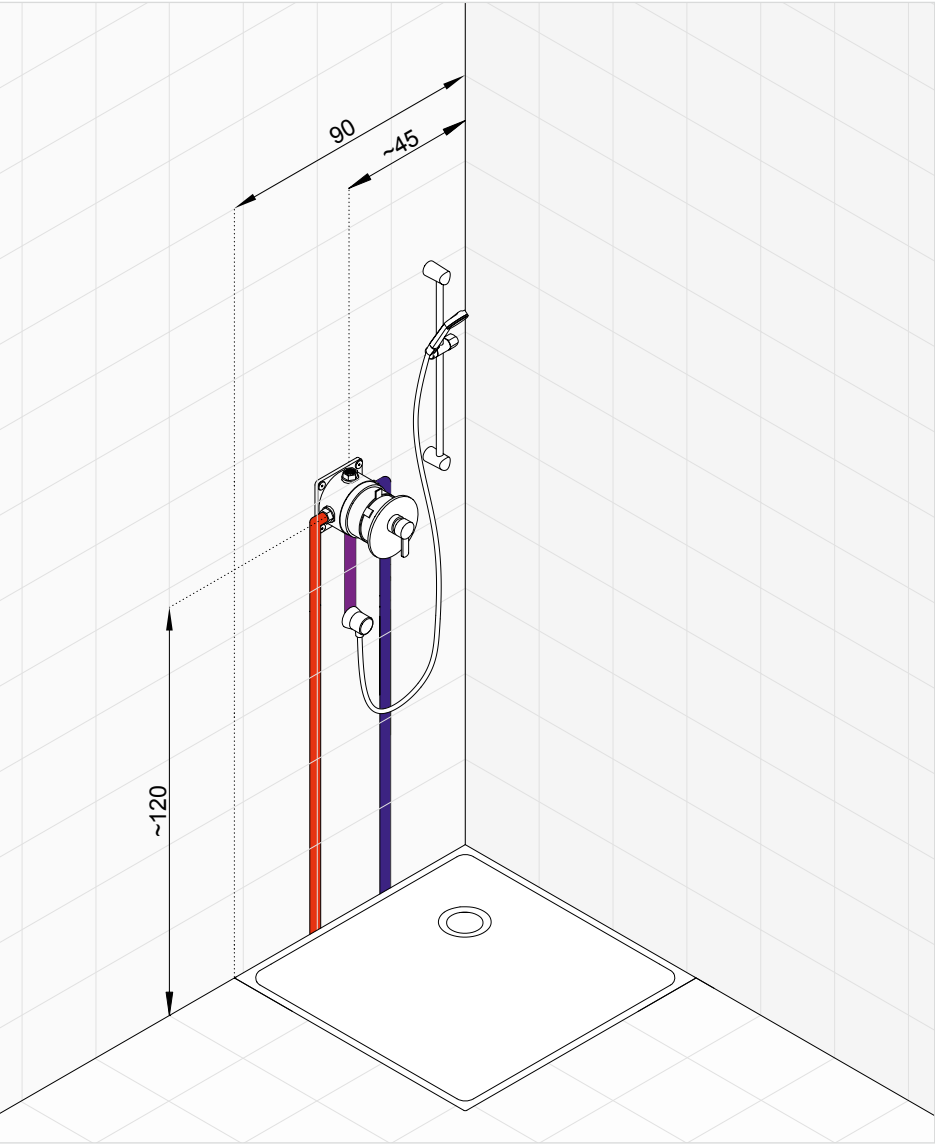
Klasický podomítkový rozvod ke sprchové sestavě.
