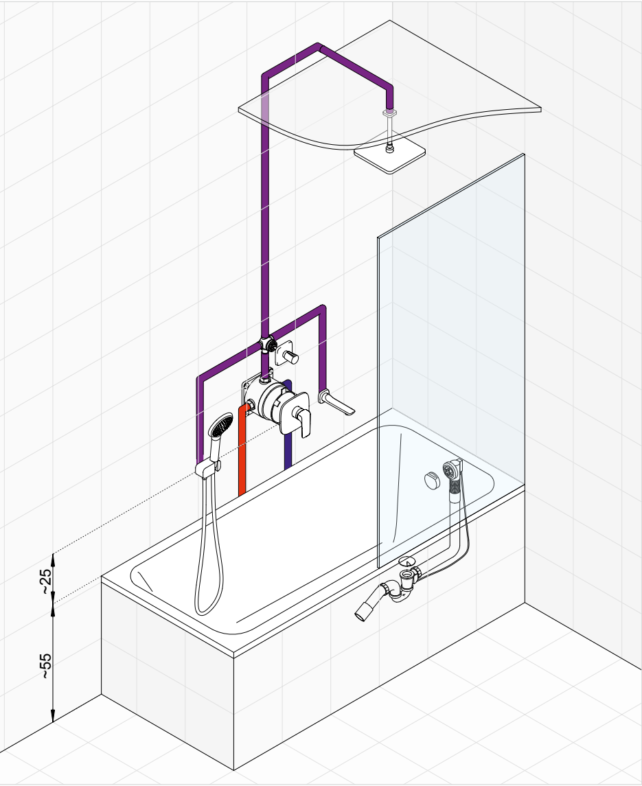
Napouštění vany nástěnným výtokem. Sprchová baterie pustí proud vody do třícestného přepínače a ten řídí tok vody mezi hlavovou sprchou, sprchovou soupravou a výtokem.
