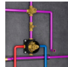
KLUDI - Instalace podomítkového rozvodu - sprcha Podomítková termostatická baterie, hlavová sprcha, boční trysky a ruční sprcha
