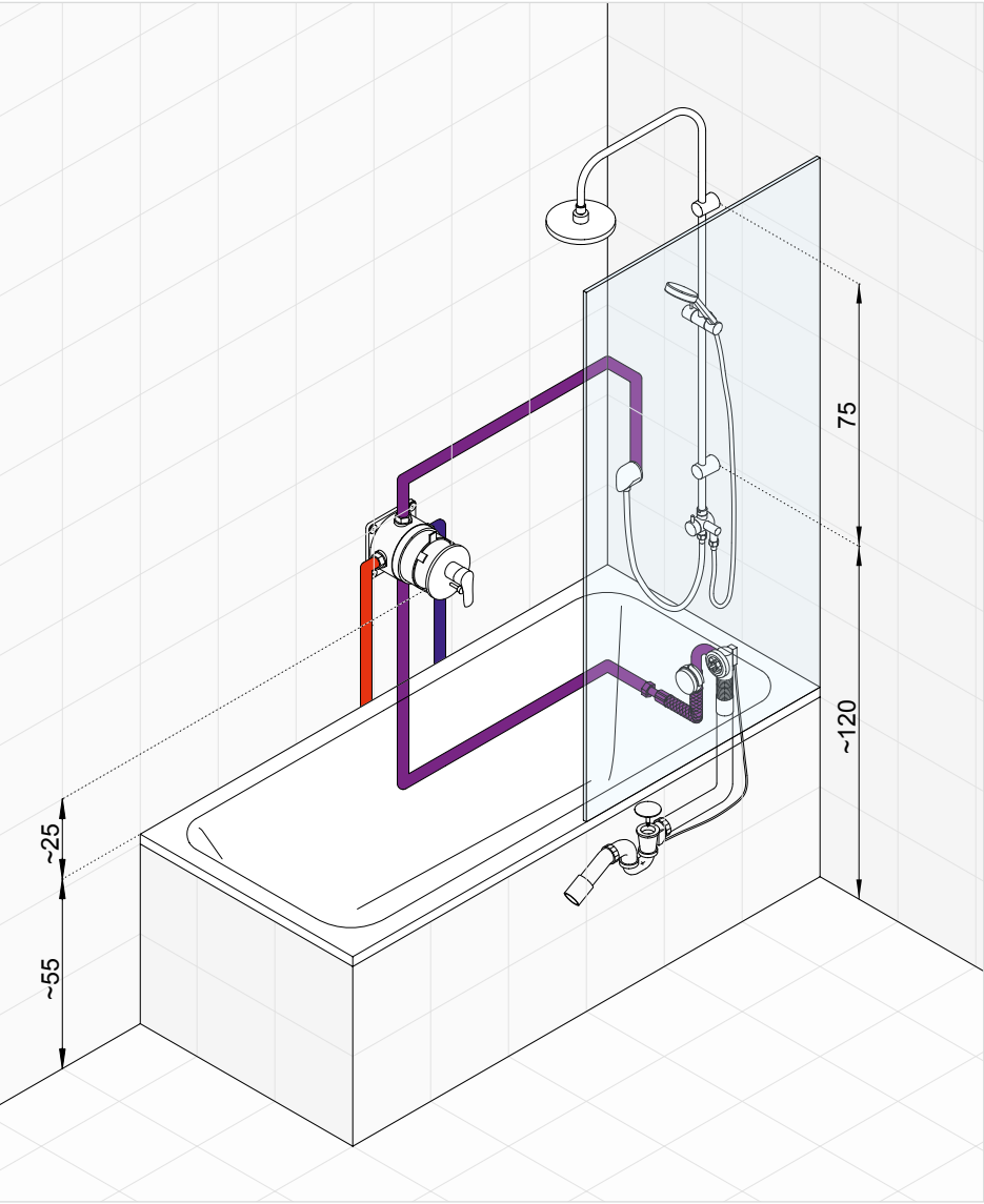
Vanová a sprchová baterie umožňuje přepínat vodu mezi napouštěním vany přepadem a KLUDI DUAL SHOWER SYSTÉMEM, který umí přepínat vodu mezi hlavovou a ruční sprchou.
