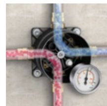
KLUDI FLEXX.BOXX Proplachování instalace
