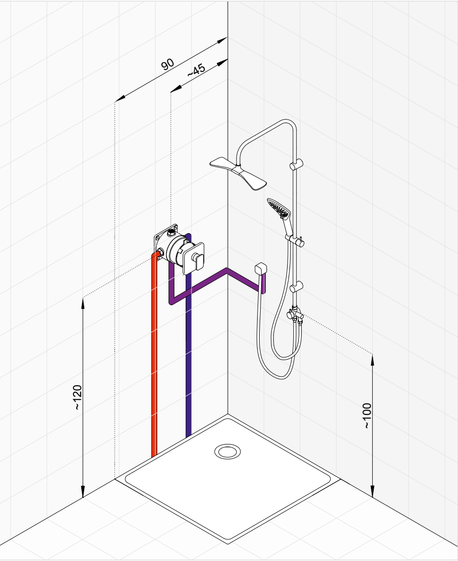
Sestava KLUDI DUAL SHOWER SYSTEM nabízí ruční a hlavovou sprchu integrovanou do jednoho setu. Voda je dodávána jednou podomítkovou vodní cestou pomocí hadicové přípojky.
